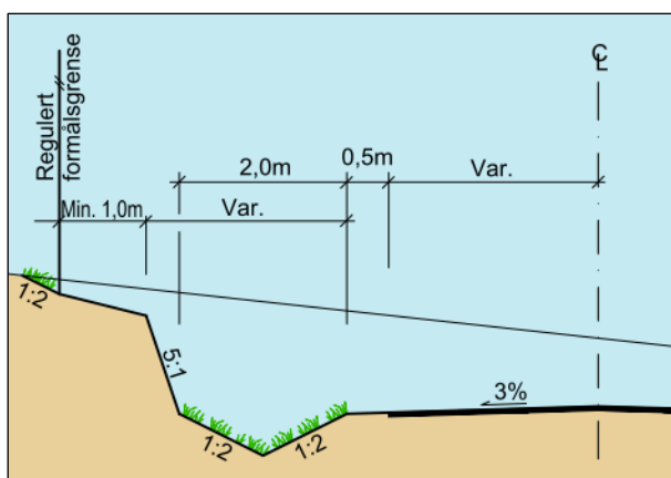
Figur 5.1: Prinsipp for reguleringsgrense ved fjellskjæring
