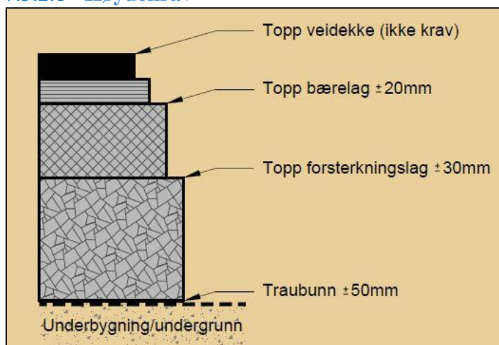
Figur 7.6: Toleransekrav i overbygningen
