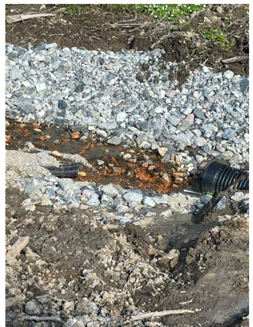
Sikring av rørutløp mot erosjon kan være et tilskuddsberettiget tiltak. Foto: Landbrukskontoret
