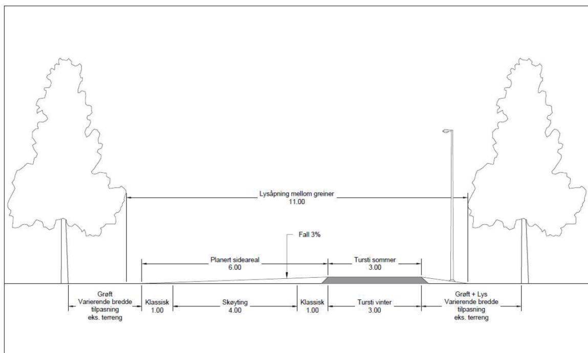
Figur 1: Forslag til snitt for lysløypetrasé vinter og sommer, turvei og planert sideareal for skiløype.
