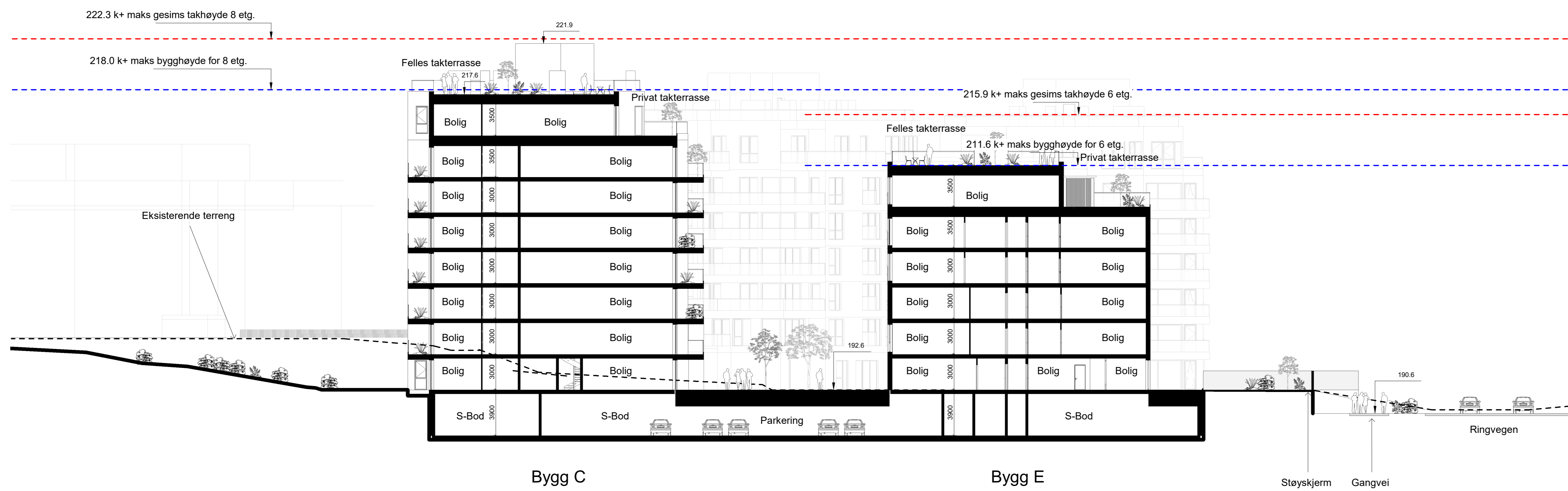
Kortsnitt A-A
