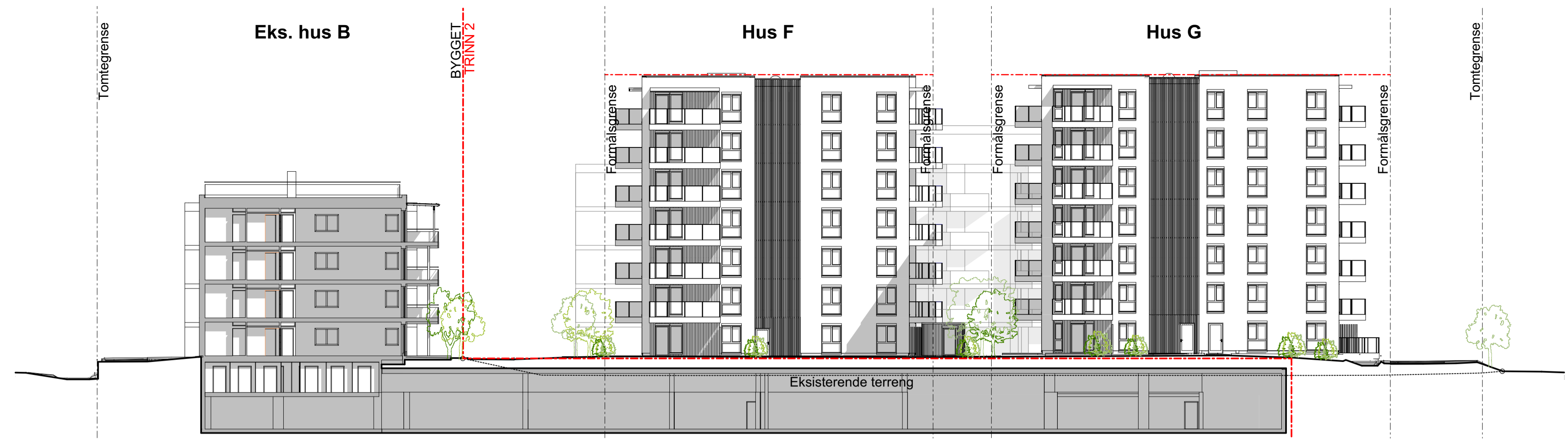
1:250 Fasade Nord
